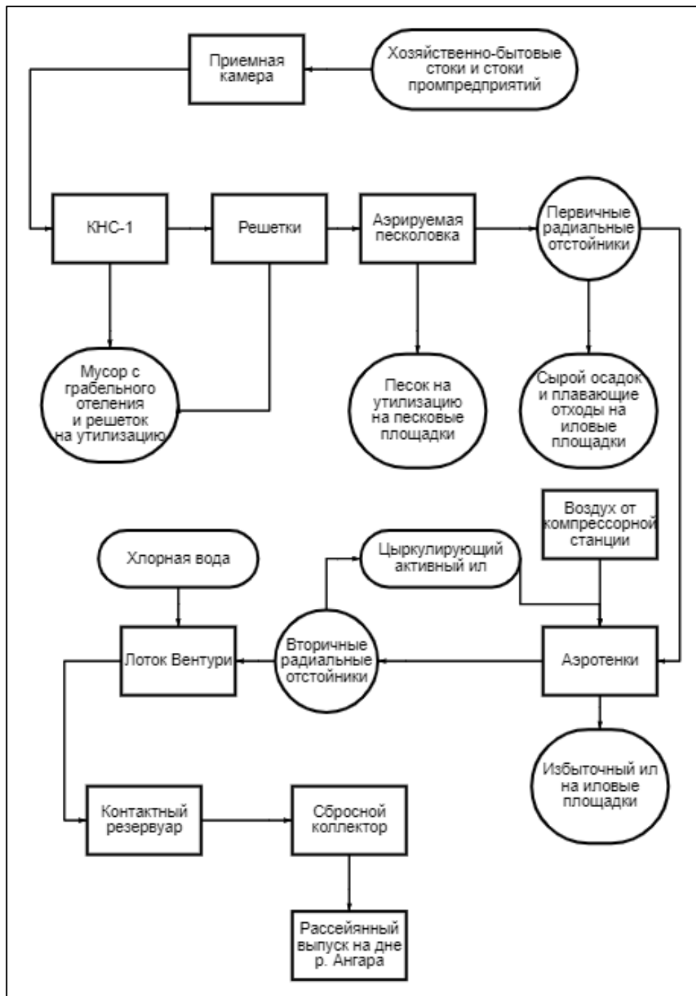
Рисунок 2.1.2. Технологическая схема КОС м.о. «город Усолье-Сибирское»
